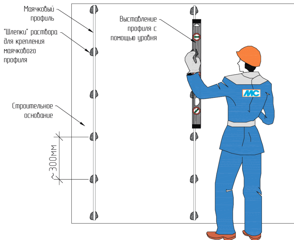
Рис.13. Монтаж маяка с помощью правила с уровнем
