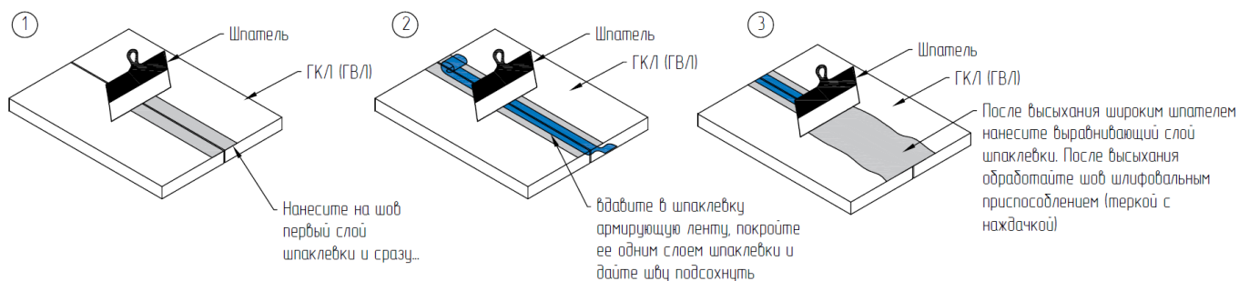
Рис. 24. Порядок шпаклевки швов между листов ГКЛ (ГВЛ) с использованием армирующей сетки
