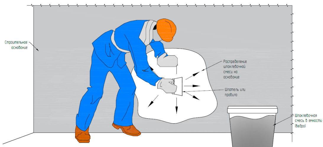
Рис. 23. Организация работ по нанесению шпаклевочной смеси
