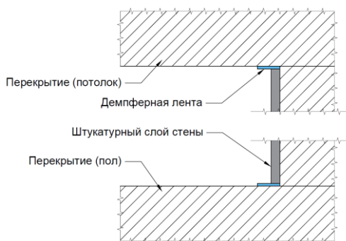
Рис.15. Приклейка демпферной ленты в местах сопряжения штукатурного слоя со стеной и потолком
