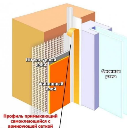
Рис.16. Профиль примыкающий с армирующей сеткой
